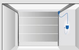
Antrieb in der rechten Torlaufschiene. Steuerung direkt neben dem Tor im Bereich des Seitenanschlags.
