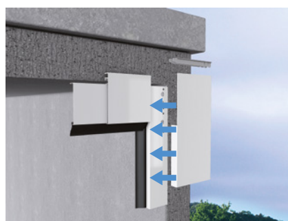
Universal-Blendenlösung, Außenansicht
